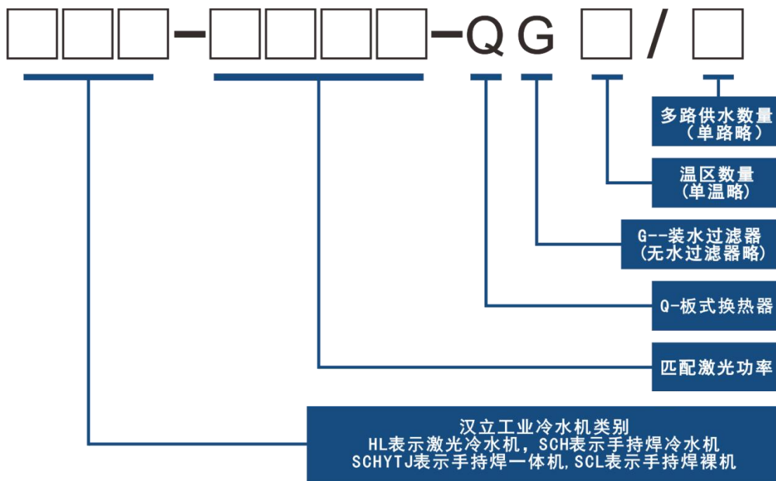
图 3-1 型号说明
