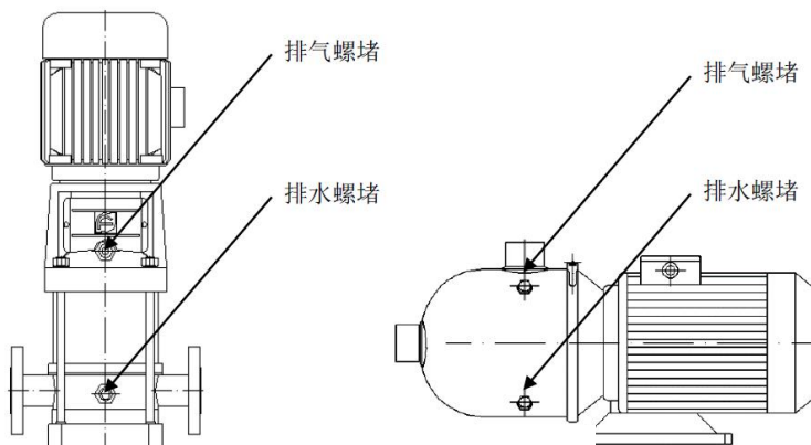
图 6-6 水泵排气与排水
