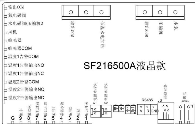
图 10-2 380V 液晶屏控制 器 电路图
