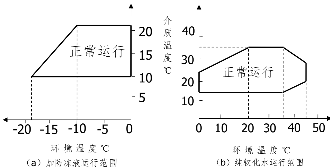
图 2-1 设备运行范围
