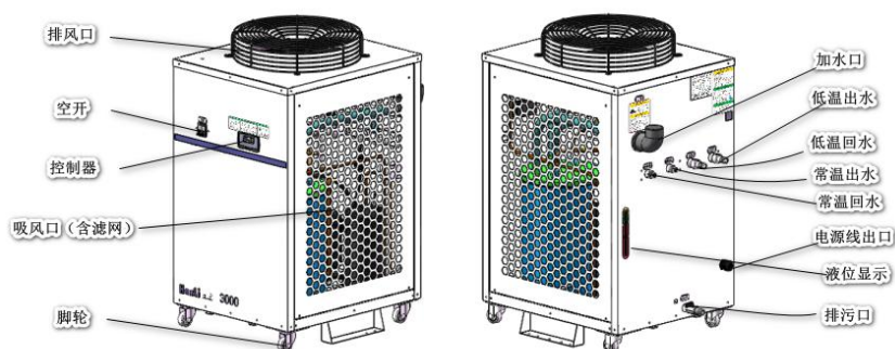
图 5-1 外形及部件名称
