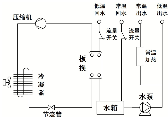
图 1-1 冷水机系统组成及工作原理
